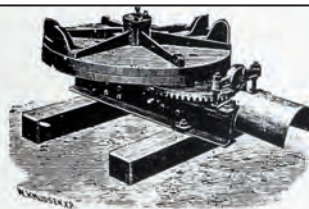
Hestevandring fra Ise Bruk, illustrasjon fra International Harvester Company's katalog nr. 54, ca. 1915.
